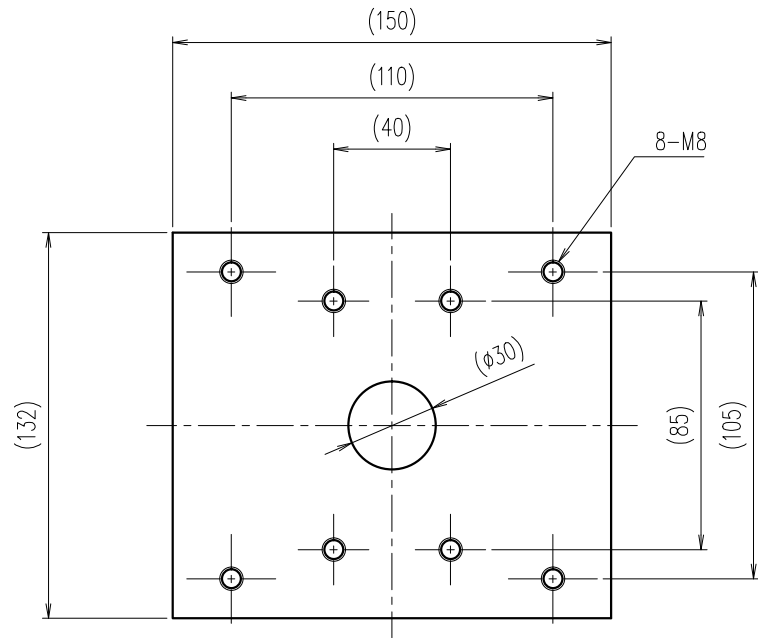
ブラケット類取付部寸法
